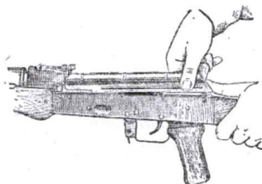
Рисунок 3. Отделение крышки ствольной коробки
