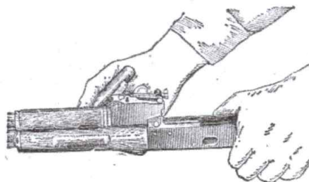
Рисунок 7. Отделение затвора от затворной рамы
