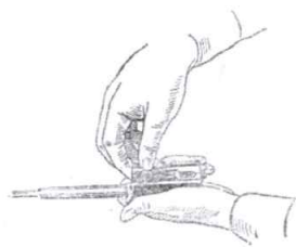
Рисунок 6. Отделение затвора от затворной рамы
