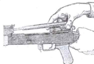
Рисунок 5. Отделение затворной рамы с затвором
